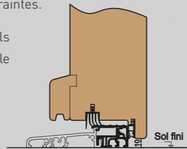
Seuil de base à rupture thermique S15-70 + joint brosse
