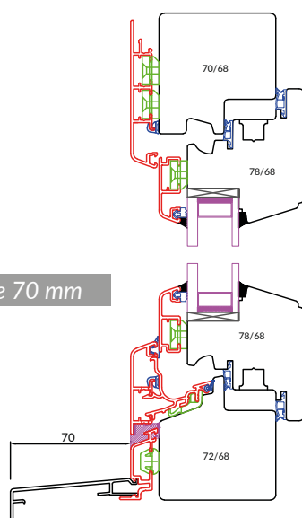
Appui bois avec habillage aluminium de 128 mm
