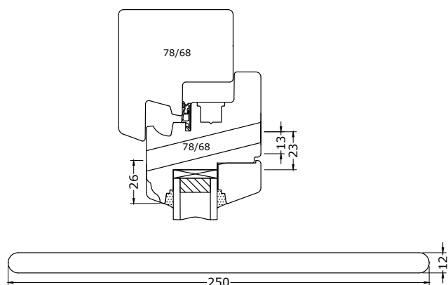
Mortaise simple ou double selon taille de la grille de ventilation
