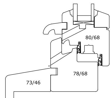
Appui élargi INOVA®
